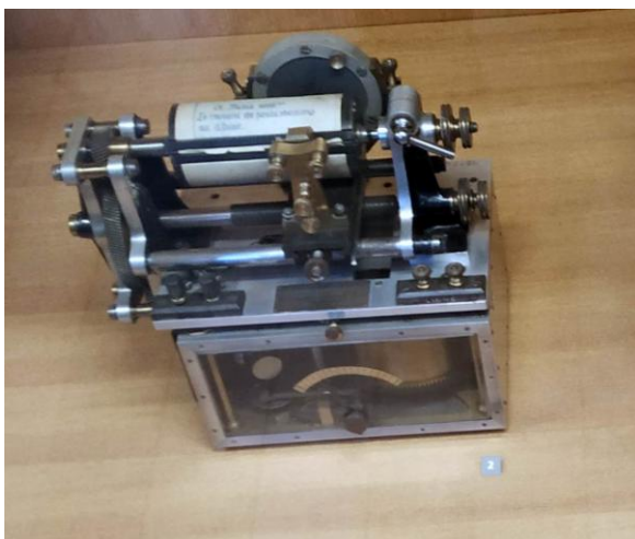
Premier appareil portable transmetteur de photoélectrographie dit « Bélinographe » 1912
